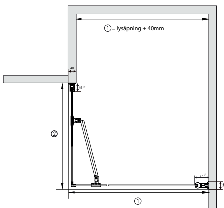
Uten magnetprofil - rett
