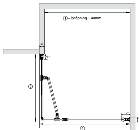
Med magnetprofil - rett
